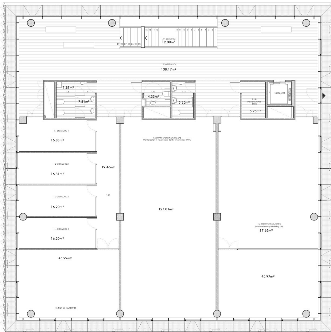
Centro UCA-SEA. Planta primera
