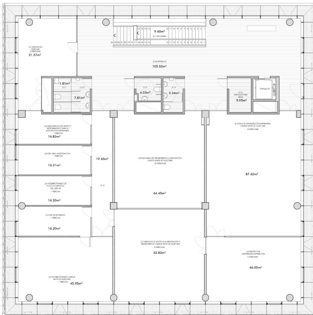
Centro UCA-SEA. Planta segunda
