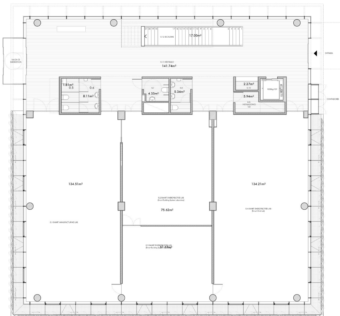
Centro UCA-SEA. Planta baja
