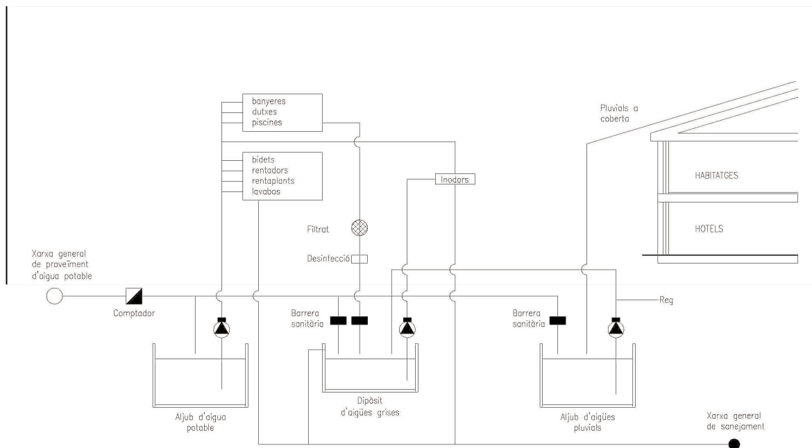
ESQUEMA D'INSTAL·LACIÓ D'AIGÜES GRISES I PLUVIALS EN HABITATGES I HOTELS
