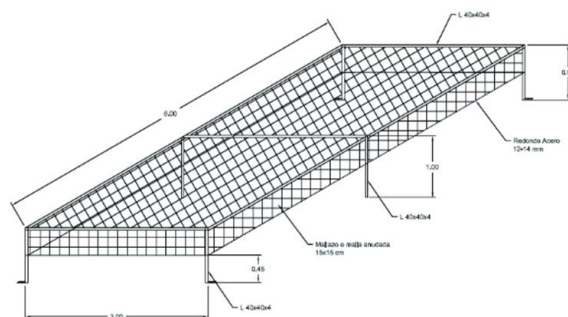
MODELO COMEDERO SELECTIVO JABALÍ
