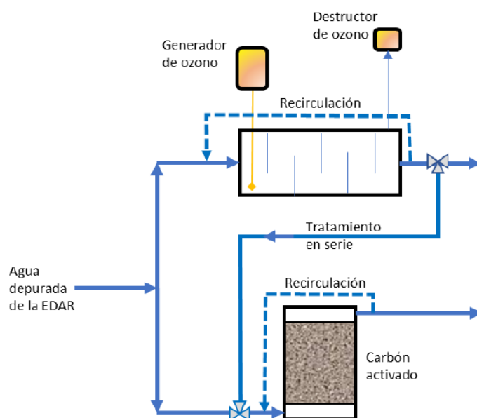
Figura 1: Esquema de tratamientos ozonización/carbón activado
